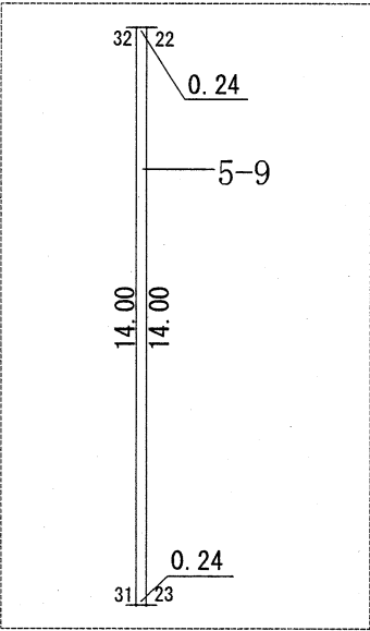
拡大図 1/200
