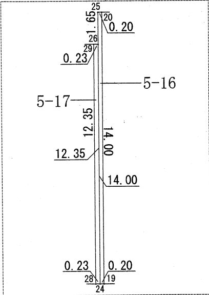
拡大図 1/200
