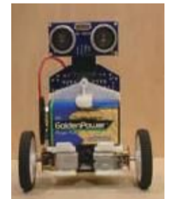
ロボットの大きさ たて約6cm よこ約8cm 高さ約10cm
