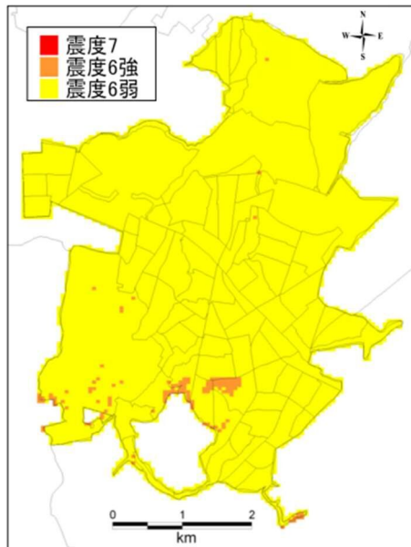
図-2 震度分布
