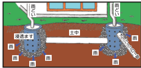
雨水が屋根から雨どいを伝って浸透ますに入り、地中へ染み込みます
