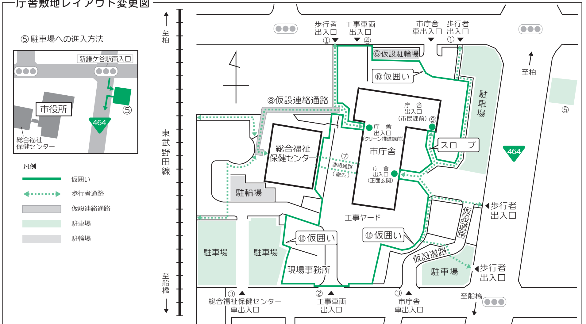
庁舎敷地レイアウト変更図
