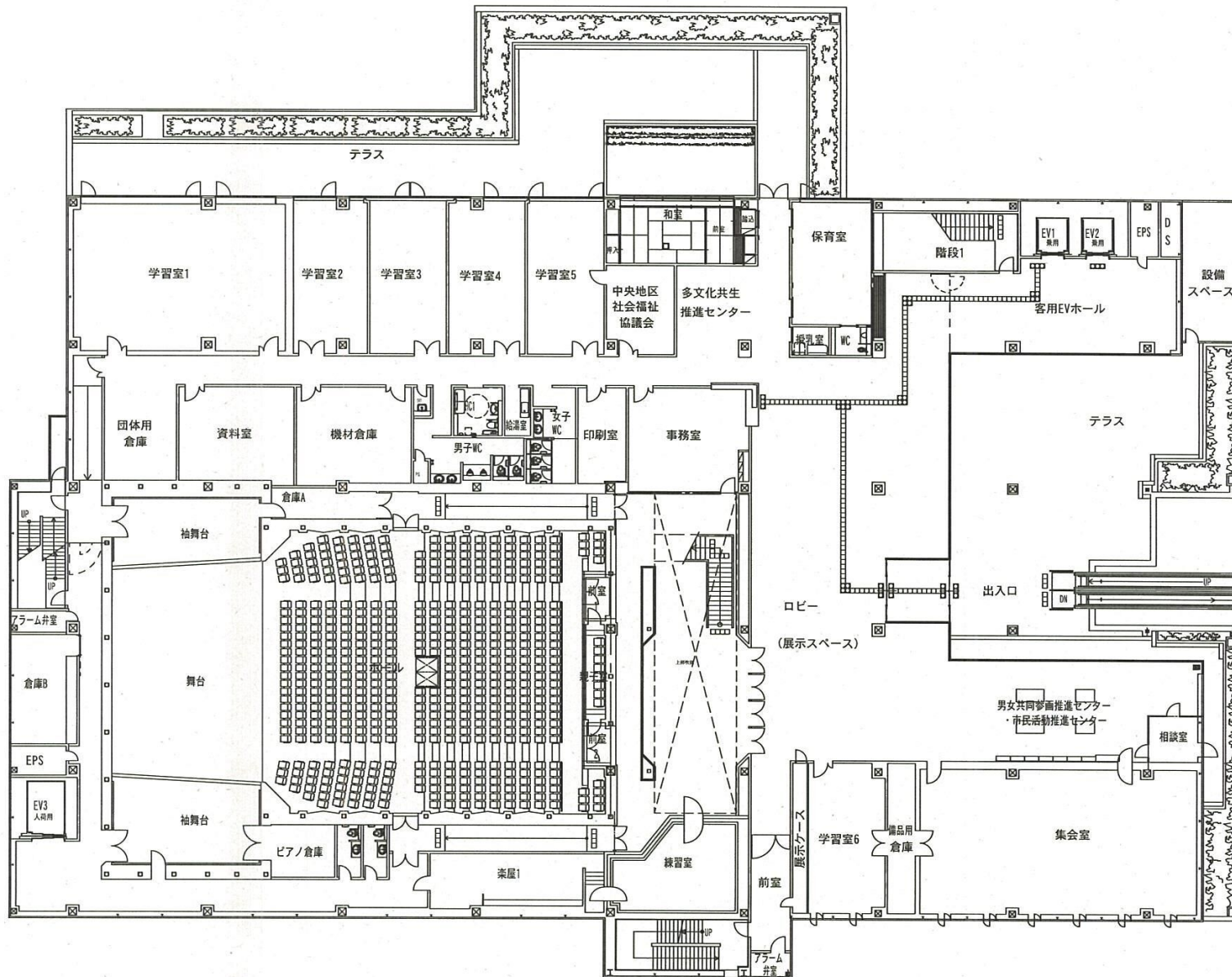
3階平面図
